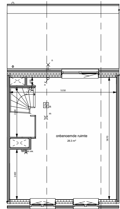
3e VERDIEPING
