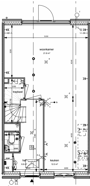
BEGANE GROND
