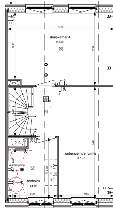
2e VERDIEPING
