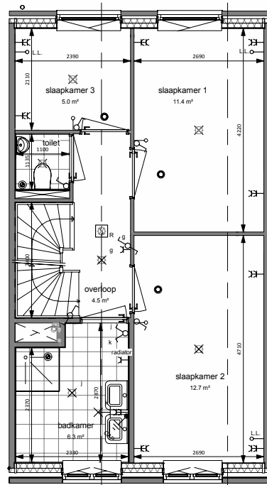
1e VERDIEPING
