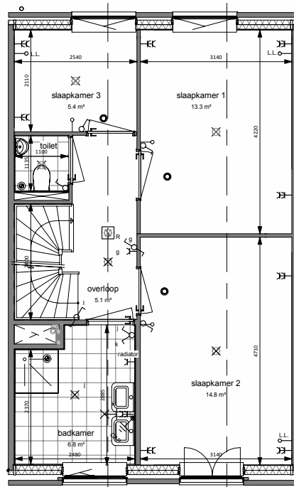
1e VERDIEPING
