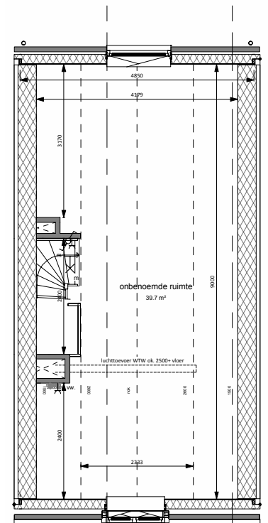
3e VERDIEPING
