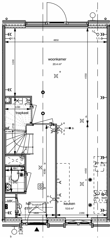
BEGANE GROND
