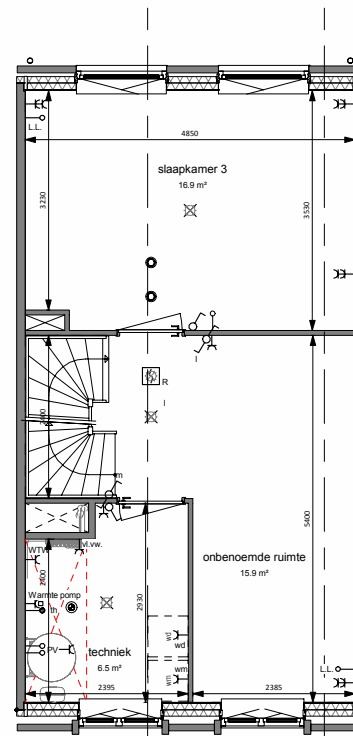
2e VERDIEPING
