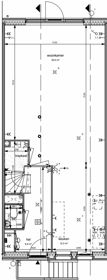
BEGANE GROND
