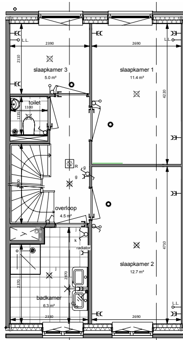
1 e VERDIEPING
