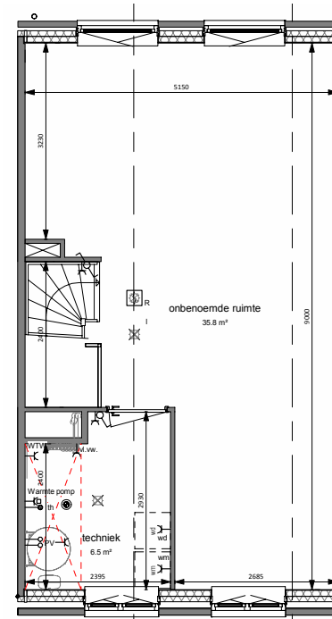
2 e VERDIEPING
