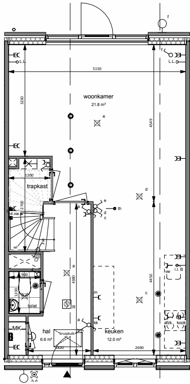
BEGANE GROND
