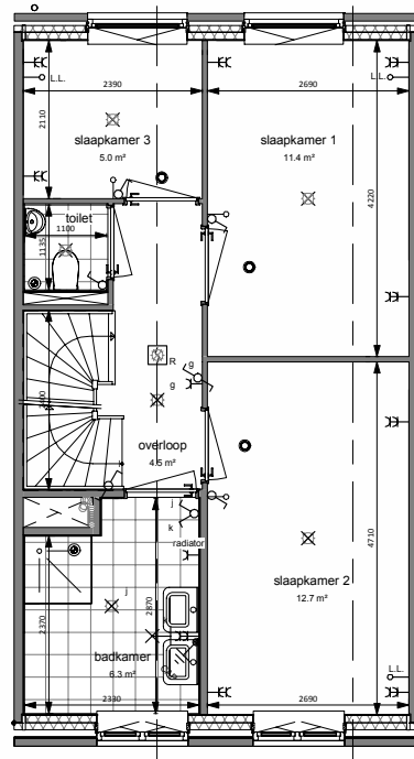
1e VERDIEPING
