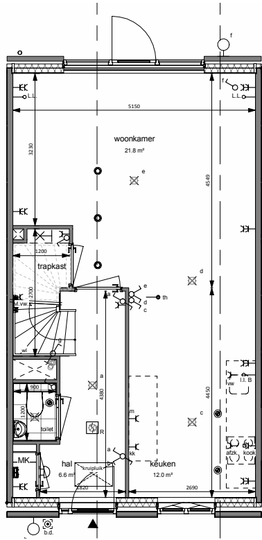
BEGANE GROND
