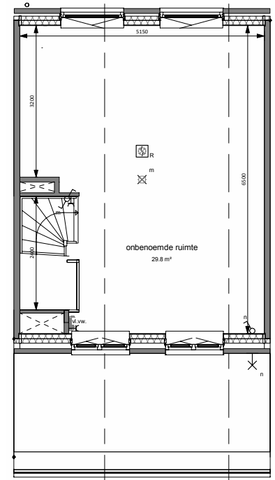
3e VERDIEPING
