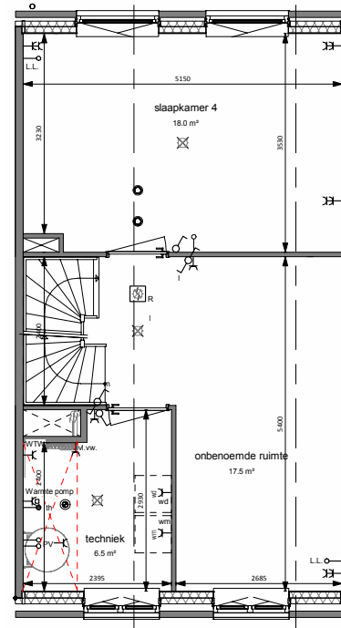
2e VERDIEPING
